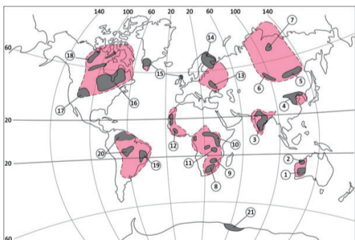
圖2 全球太古宙克拉通(cratons)的分布(灰色區塊)，其中粉紅色區塊一般認為是上伏的太古宙-元古宙之地塊(terraces)。
