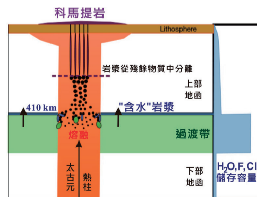
圖6 太古宙地函熱柱上湧通過地函過渡帶，周圍的礦物相變而釋放流體，助長了地函熱柱的熔融作用(圖示中，原有的小黑點變成大黑點)。
