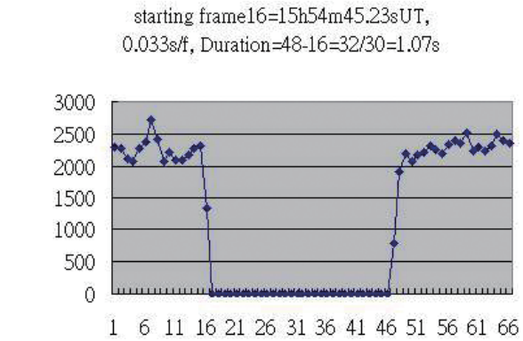
圖2 典型的掩星光度變化圖，此圖是2006年12月27日晚上所觀測到的1438號小行星(Wendeline)掩HIP 38332號恆星。(林志隆提供)
