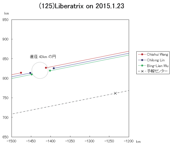
圖3 這是2015年1月23日本館研究人員和臺中一中的王家輝老師以及在彰化觀測的吳炳連老師分別觀測到的125號小行星(Liberatrix)掩星結果，把資料彙報到薩摩川內市せんだい宇宙館後，由早水勉先生繪製成本圖。(早水勉提供)
