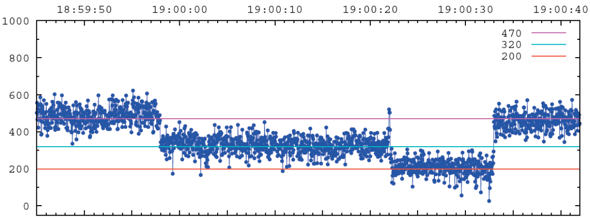
圖1 2006年10月18日(UT)晚間在臺中觀測到的84號小行星掩SAO 80166號恆星的光度變化圖。這樣的特徵通常表示被掩恆星其實不只一顆，而是多重恆星系統。同時間鹿林天文臺則沒有看到這樣的兩段式減光現象。(林志隆提供)
