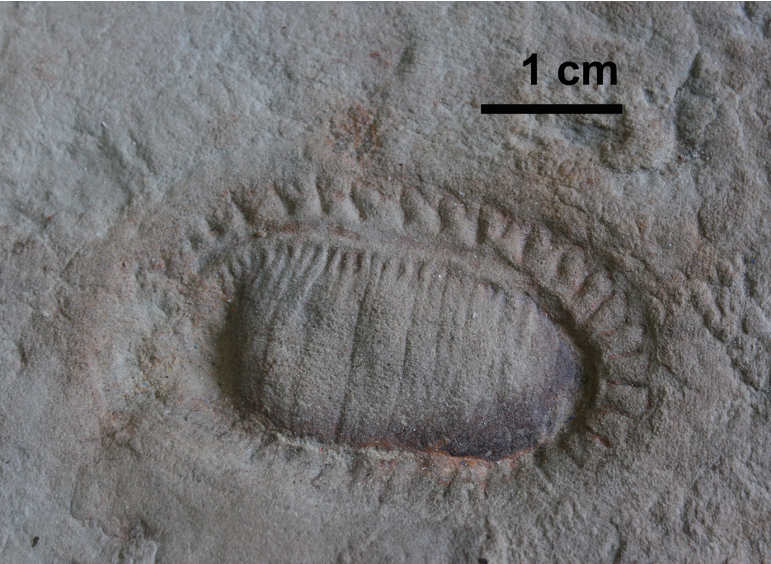
圖4 金伯拉蟲(Kimberella), 產自俄羅斯的白海。
