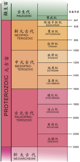
圖1 元古宙的地質年代
