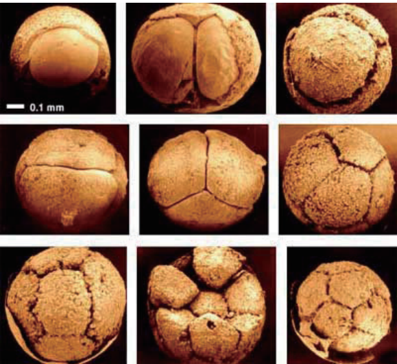
圖2 陡山沱層的胚胎化石(取自Prof. Shuhai Xiao, Virginia Tech Univ的網站)
