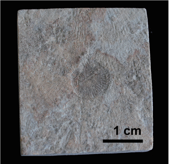
圖5 狄氏水母(Dickinsonia), 產自俄羅斯的白海。
