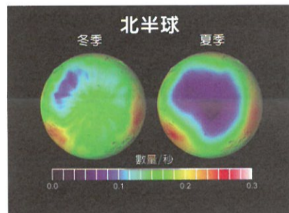
圖5. 火星奧德塞探測船所拍攝，在火星北半球夏、冬季節時冰帽的變化。
