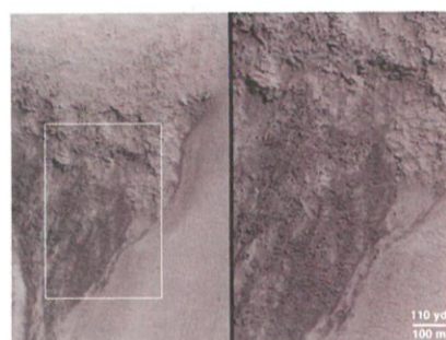
圖2. 在火星坑壁上的細微照片，似乎可見類似地球土石流的痕跡。右圖是左圖白色方塊的放大。
