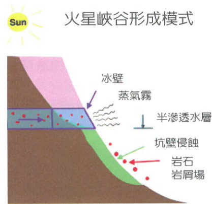
圖3. 火星峽谷及隕石坑壁液態水侵蝕示意圖，圖中可見液態水層受外力作用向外噴出，而形成侵蝕及在下游處形成堆積。
