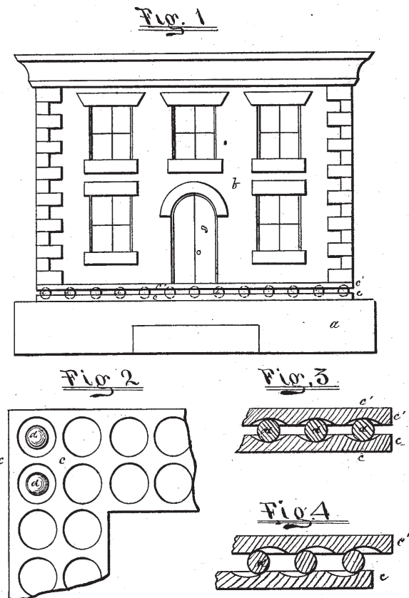
圖3 建築「曲面滑動」隔震概念。Fig.2為隔震層橫面，Fig.3和Fig.4為隔震層立剖面。摘自美國專利US99973A，發明人：Jules Touaillon，日期：1870年2月15日。
