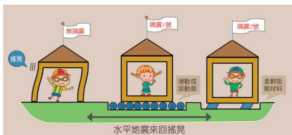
圖1 建築隔震方法和效果略圖
