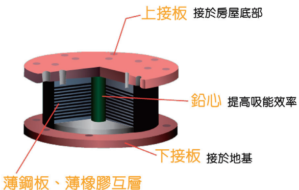
圖4 積層鉛心橡膠支承(LRB)隔震器內部構造略圖與功能說明
