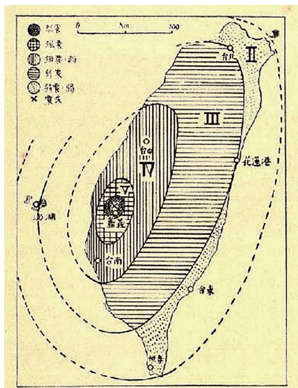
圖1 1906年梅山地震等震度圖(臺北觀測所, 1936; 鄭世楠資料)
