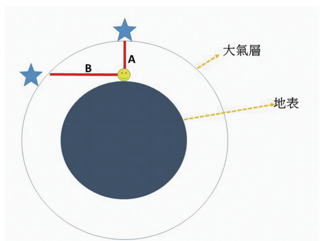
圖2 這示意圖能讓你同樣的星光在天頂的時候經過的大氣途徑(A)比較短，受到消光的影響比較少；從水平方向比較長(B)受到的影響比較大。
