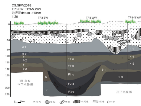
圖2 灰坑的剖面繪圖
